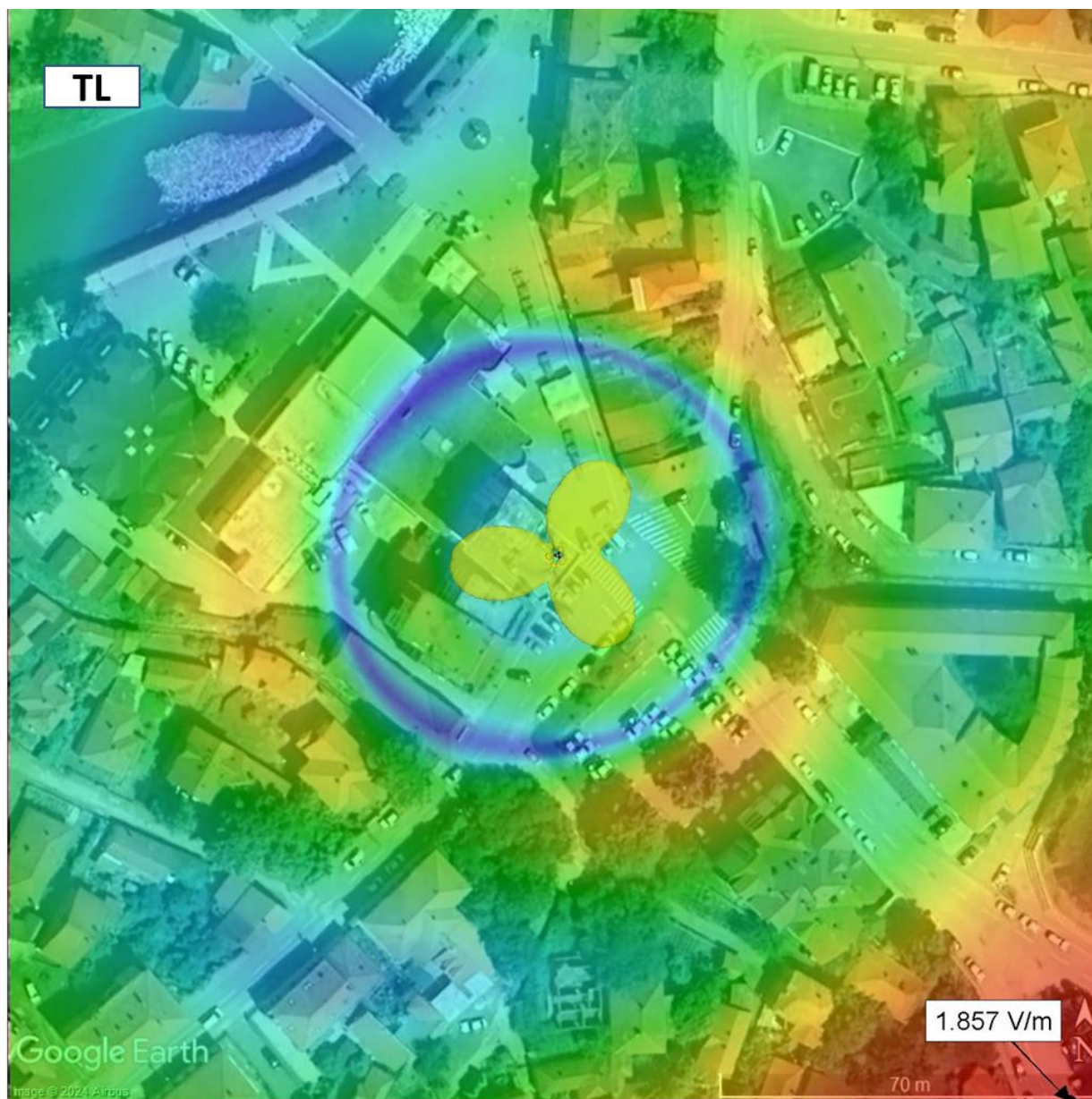
Слика 5.4. Јачина електричног поља на тлу, на јавном подручју, када радио-систем LTE800 оператора Telekom Srbija ради макс. капацитетом
