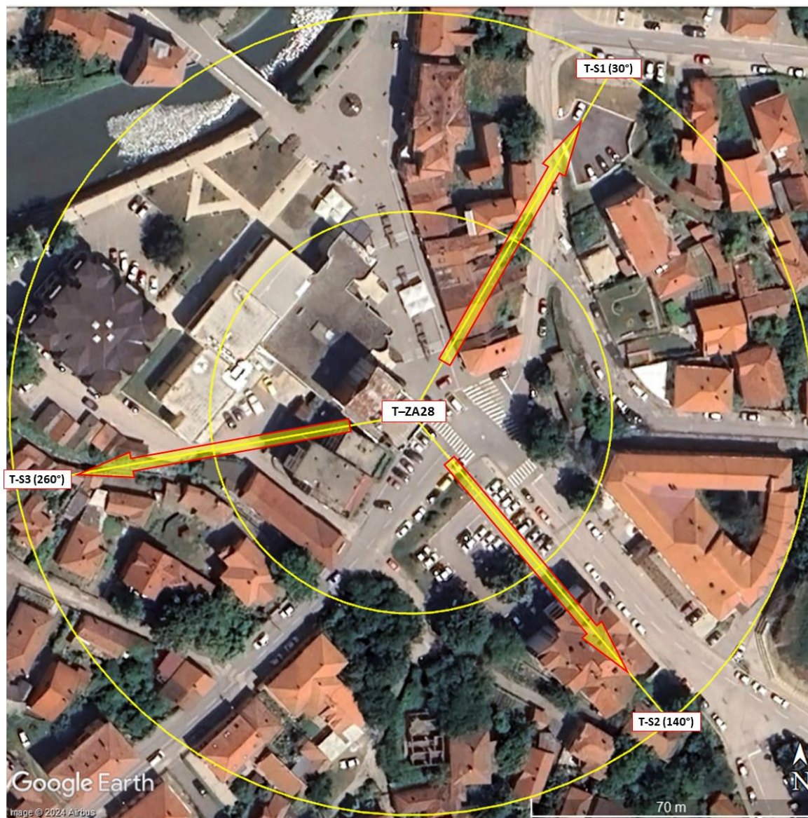
Слика 6.3. Смерови зрачења антенског система предметне РБС (са Google Earth)
