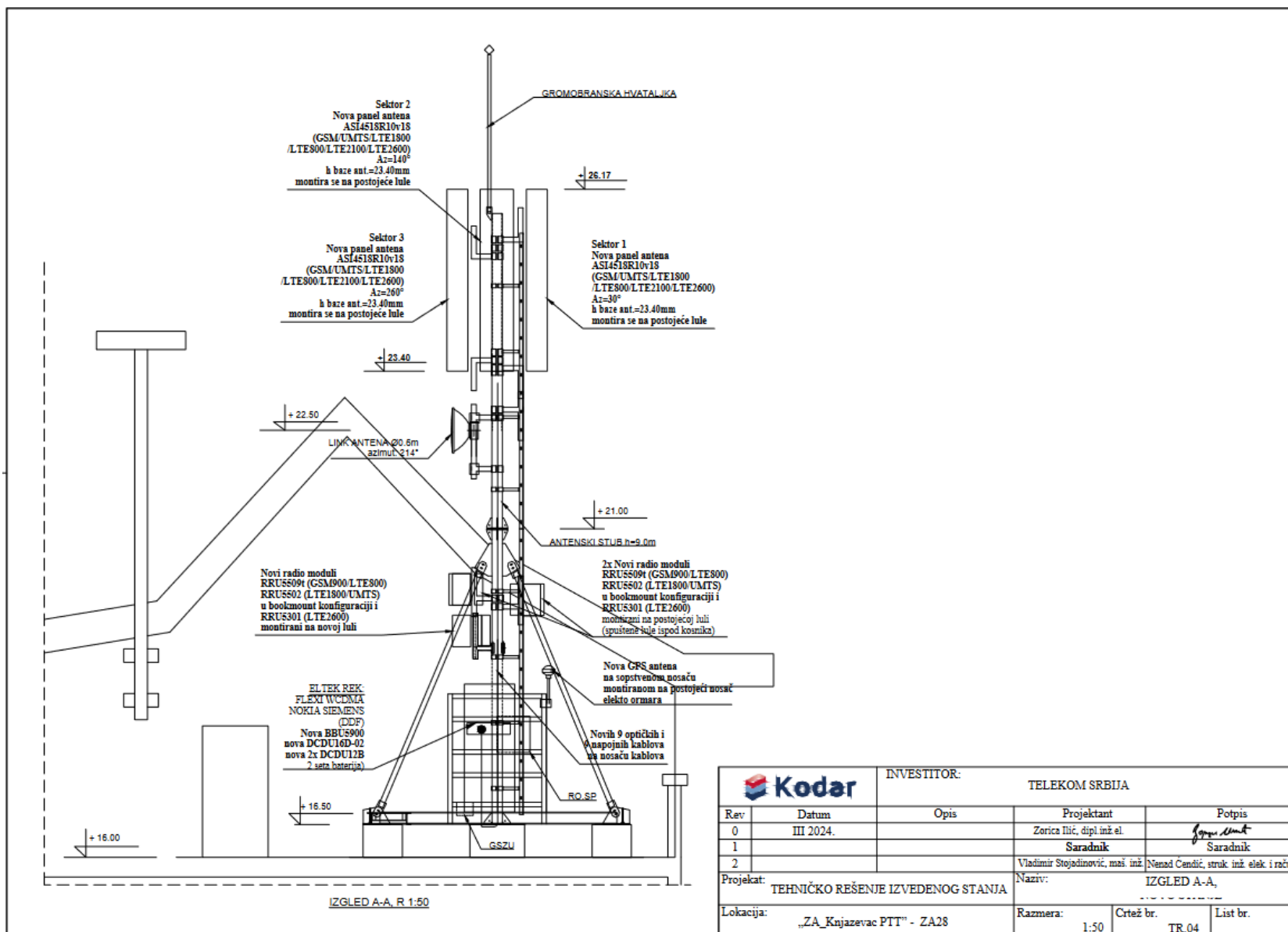
Слика 3.2. Техничко решење изведеног стања – изглед А-А
