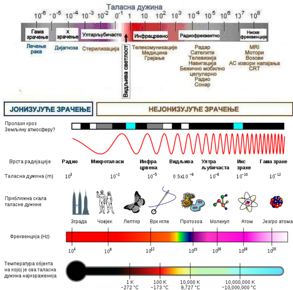
Слика 5.1. Графички приказ електромагнетног спектра (преузето са https://sr.wikipedia.org/wiki/Nejonizujuće_zračenje )
