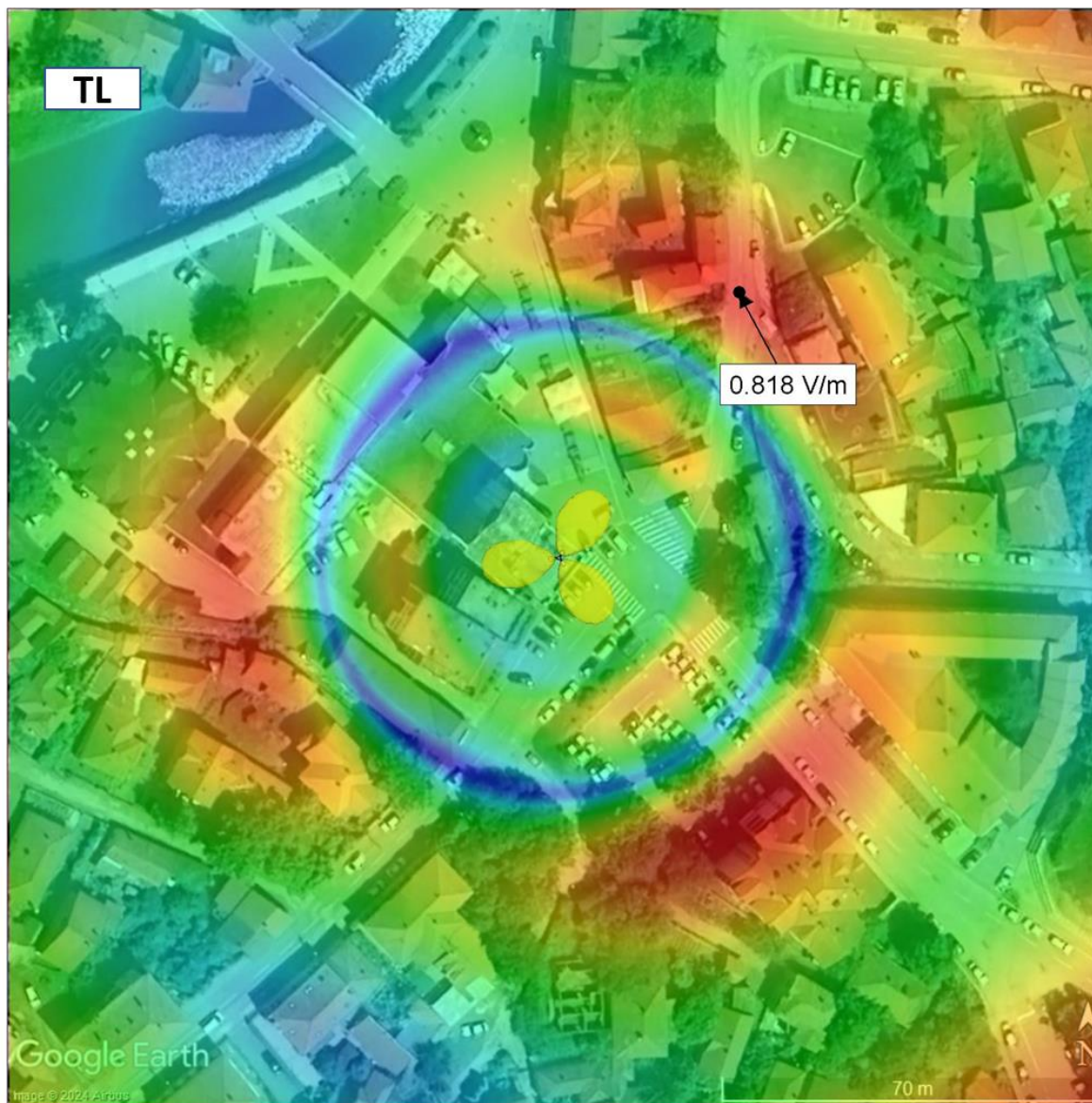
Слика 5.2. Јачина електричног поља на тлу, на јавном подручју, када радио-систем GSM900 оператора Telekom Srbija ради макс. капацитетом
