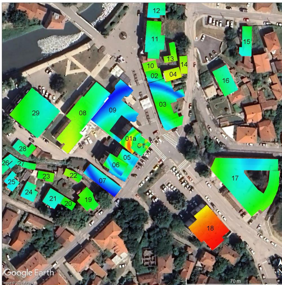
Слика 5.8. Јачина електричног поља унутар објеката када радио-систем GSM900 оператора Telekom Srbija ради максималним капацитетом
