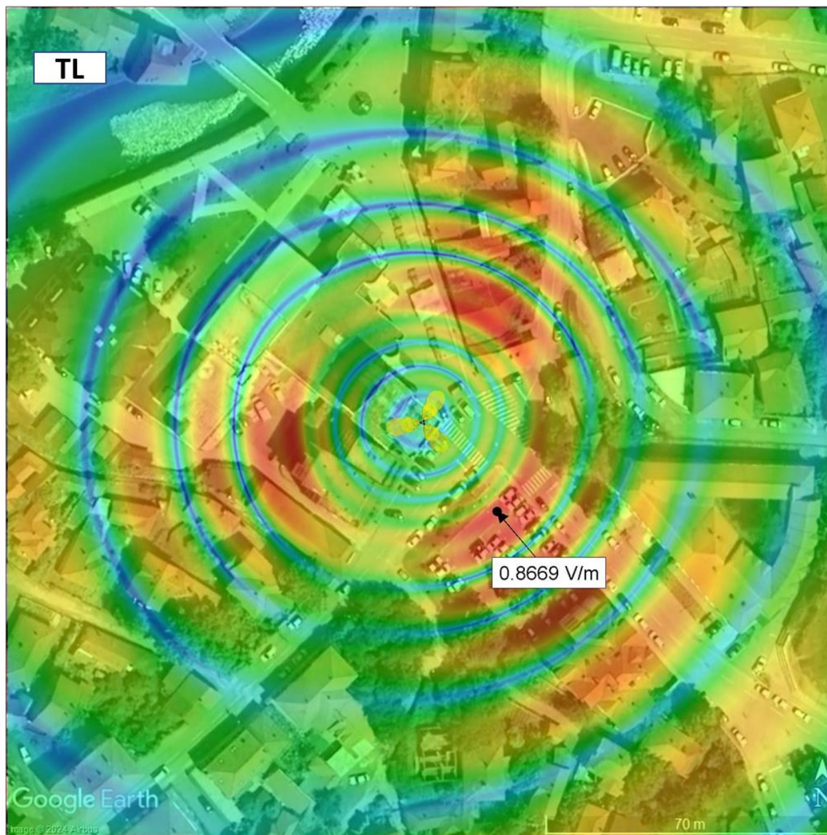
Слика 5.6. Јачина електричног поља на тлу, на јавном подручју, када радио-систем LTE2100 оператора Telekom Србија ради макс. капацитетом
