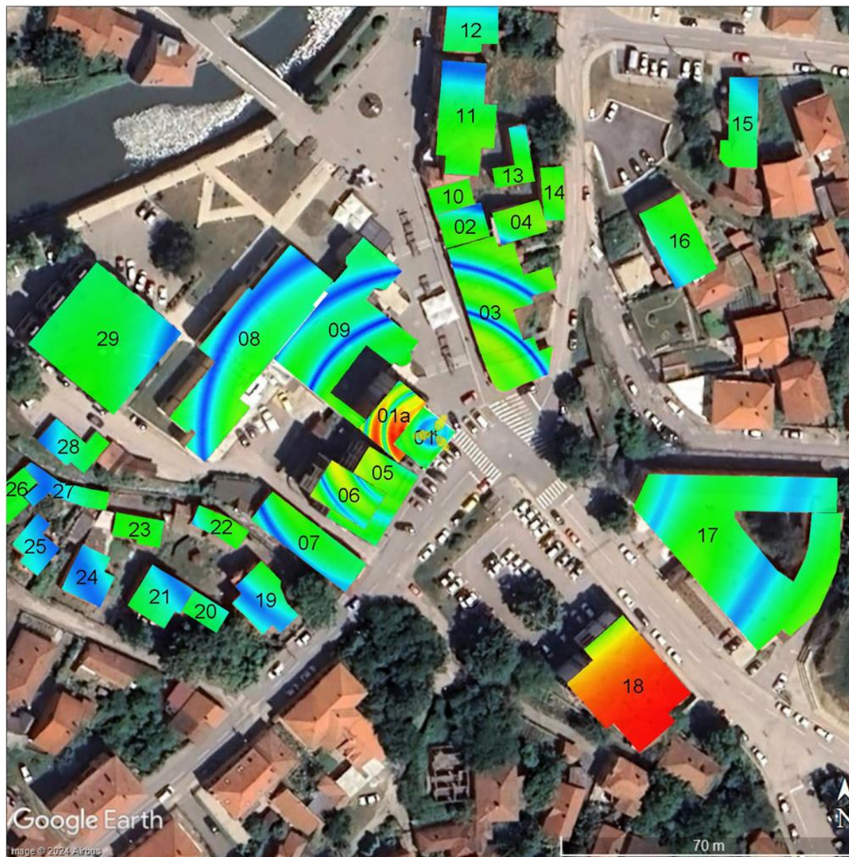
Слика 5.11. Јачина електричног поља унутар објекта када радио-систем LTE1800 оператора Telekom Srbija ради максималним капацитетом
